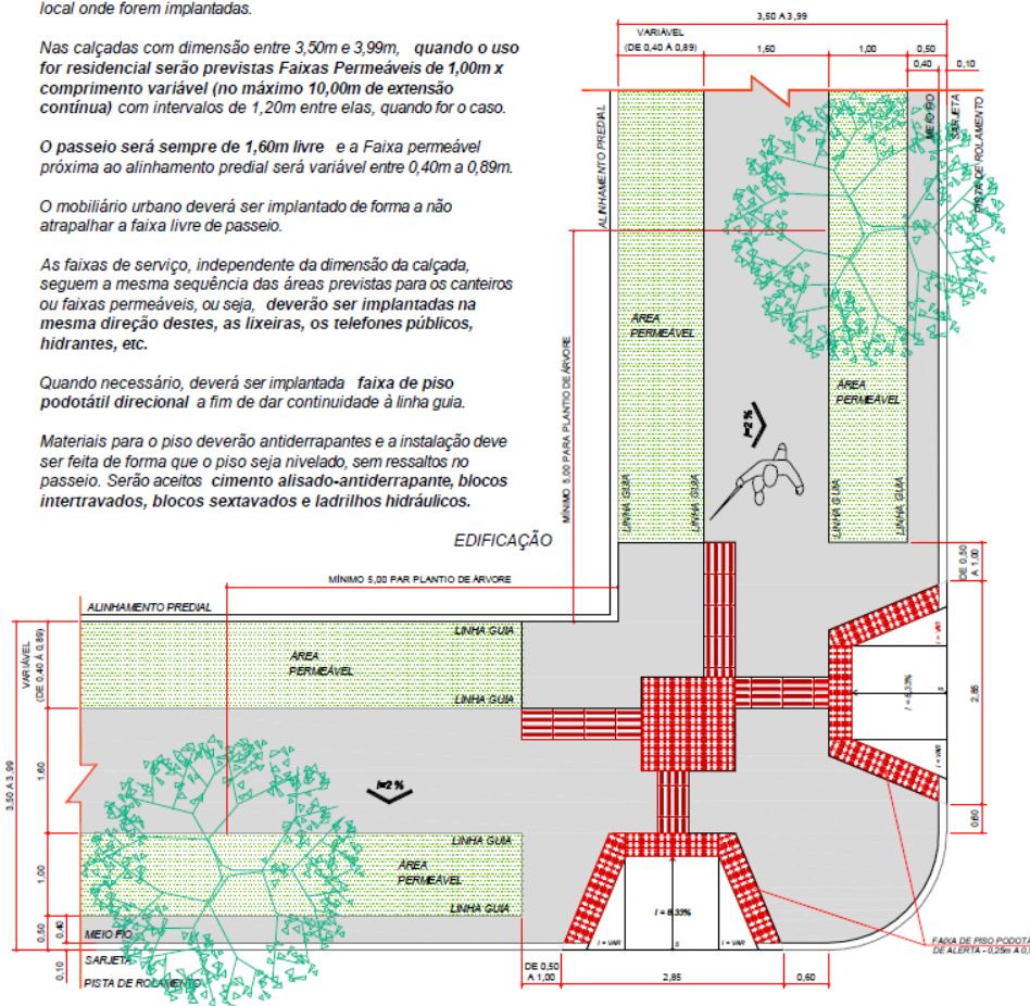
FIGURA XXX - PLANTA BAIXA - RAMPA DE TRANSIÇÃO PARA CALÇADAS DE 3,50m A 3,99m
