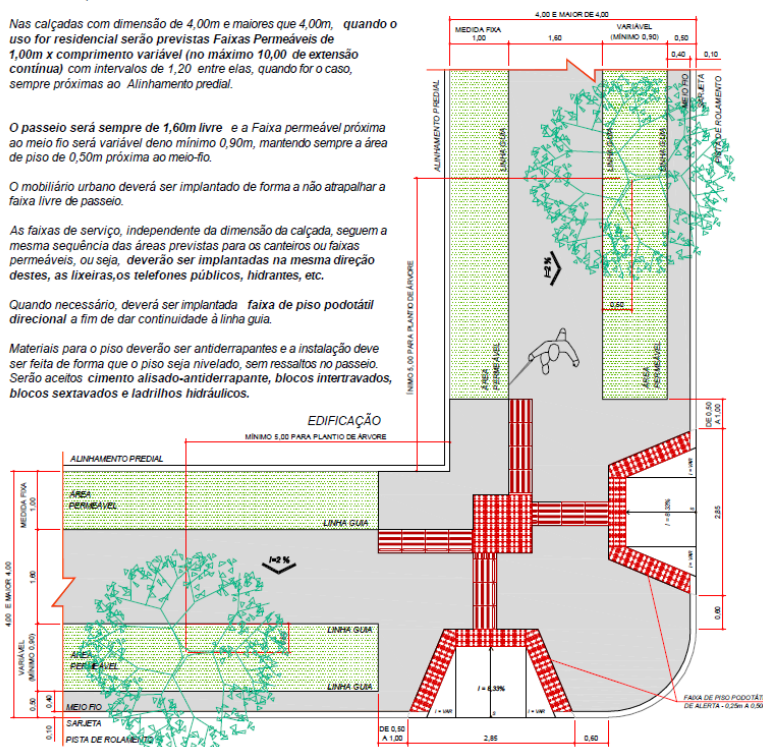
FIGURA XXXIV - PLANTA BAIXA - RAMPA DE TRANSIÇÃO PARA CALÇADAS DE 4,00m E MAIORES QUE 4,00m
