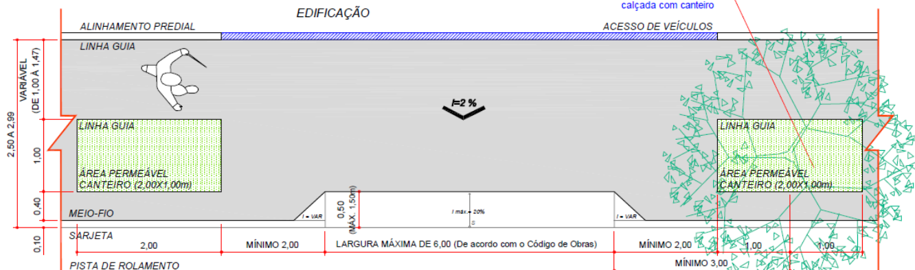
FIGURA XXIV- PLANTA BAIXA - RAMPA DE ACESSO DE VEÍCULOS PARA CALÇADAS DE 2,50m ATÉ 2,99m- Independente de a Edificação ser Residencial ou Comercial utiliza-se canteiro de 2,00x1,00m(CALÇADA CHEIA)
