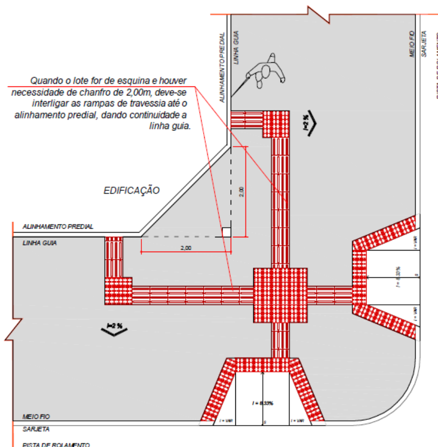
FIGURA XXXVII - DETALHES GENÉRICOS RAMPA DE TRAVESSIA E INTERSEÇÕES
