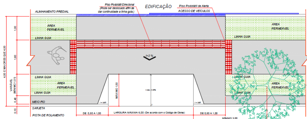
FIGURA XXXVII - DETALHES GENÉRICOS RAMPA DE TRAVESSIA E INTERSEÇÕES
