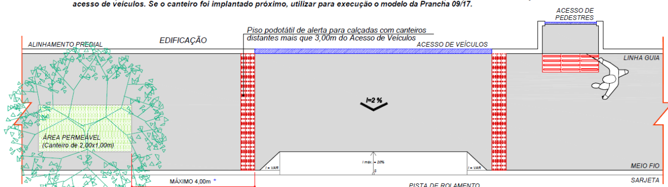
FIGURA XLII - MODELO DE PISO PODOTÁTIL DE ALERTA EM ACESSOS DE VEÍCULOS COM CANTEIROS DISTANTES
