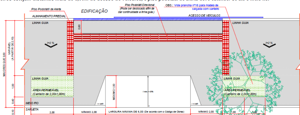
Caso os canteiros estejam distantes mais de 5,00m do acesso de veículos, o piso podotátil de alerta deve estender-se até o meio fio.
