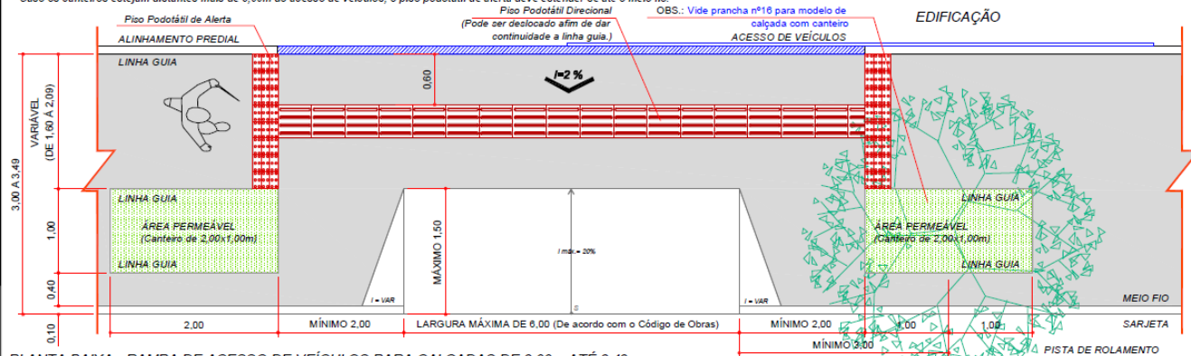
FIGURA XXIX - PLANTA BAIXA - RAMPAS DE TRANSIÇÃO PARA CALÇADAS DE 3,00m A 3,49m – Uso comercial
