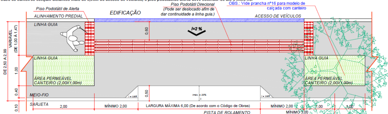
FIGURA XXV- PLANTA BAIXA - RAMPA DE ACESSO DE VEÍCULOS PARA CALÇADAS DE 2,50m ATÉ 2,99m
