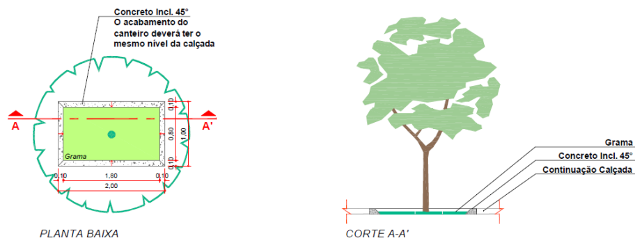
FIGURA XXXV - DETALHE CANTEIRO 2,00m x 1,00m
