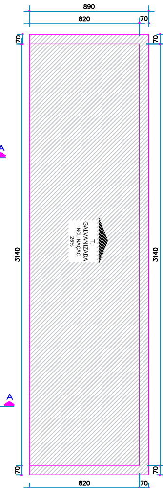
COBERTURA ESCALA / 1:100
